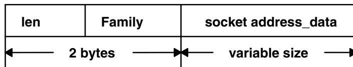
sockaddr Structure
